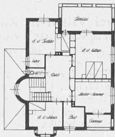
Abb. 2 bis 5. Grundrisse und Schnitt der Villa Werdmüller. — 1 : 400.
