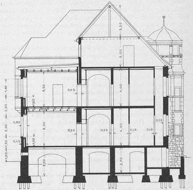
Abb. 3. Schnitt. — Masstab 1 : 200.
