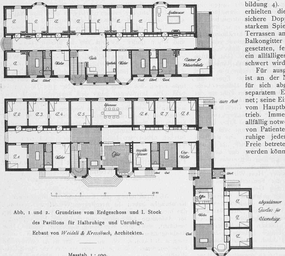
Masstab 1 : 400.
