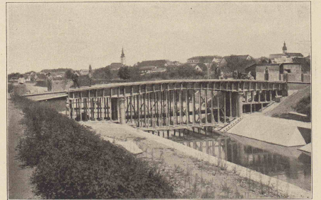
15. Brücke über die Petronyca (Oesterreich)
