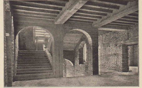
16. Schulhaus in Wollishofen-Zürich. Ansicht der Decken mit Treppenkonstruktion. Ausgeführt ca. 3000 m 2 Decken
