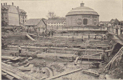
10. Hotel „Eden au Lac“ in Zürich. Die Fundation während der Ausführung
