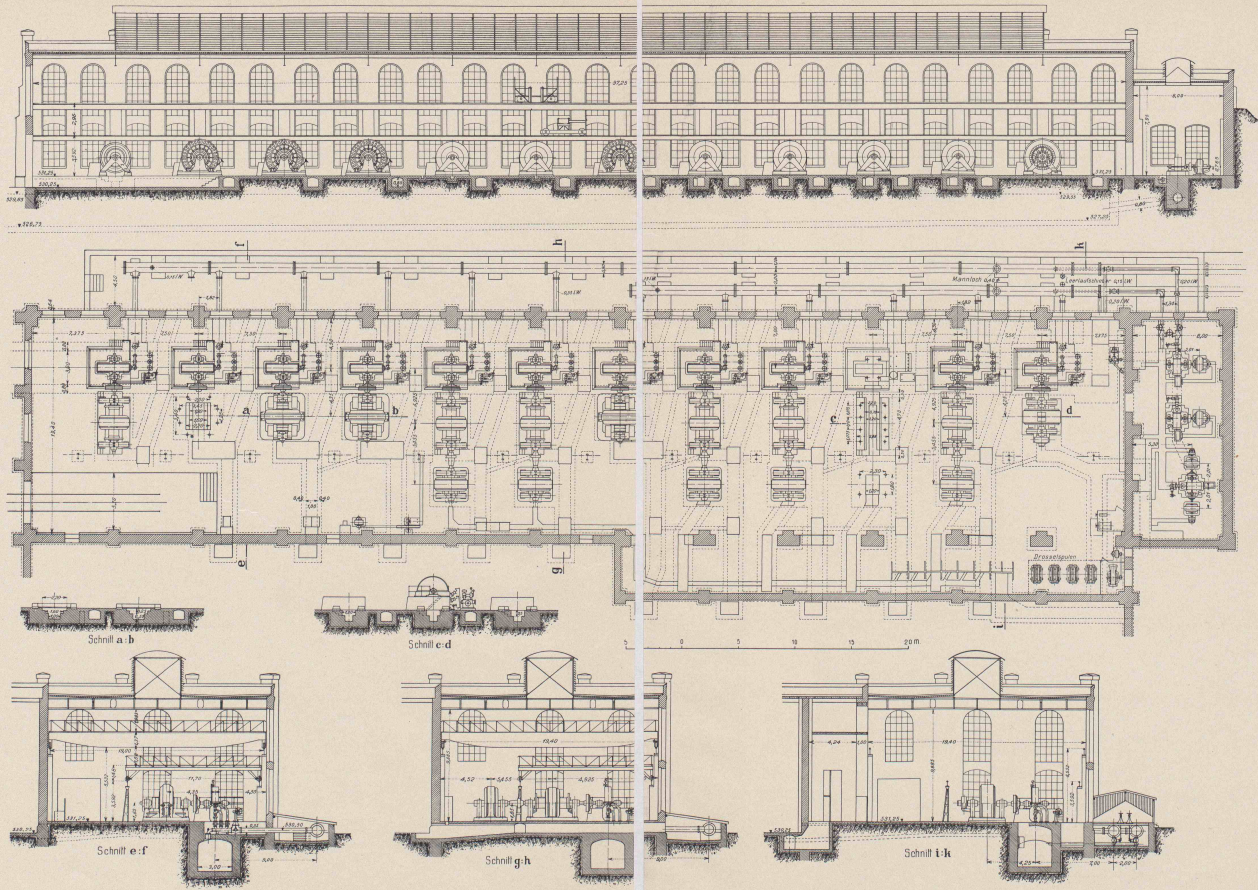
Grundriss und Schnitte
