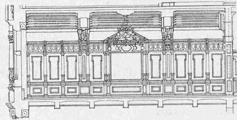
Abb. 9. Schnitt durch den grossen Saal. — 1:150.
