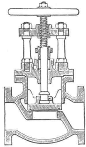
Stahlguss-Ventile mit Patentedichtung.
