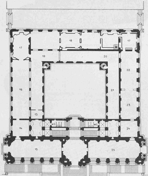
Abb. 3. Hauptgeschoss.
