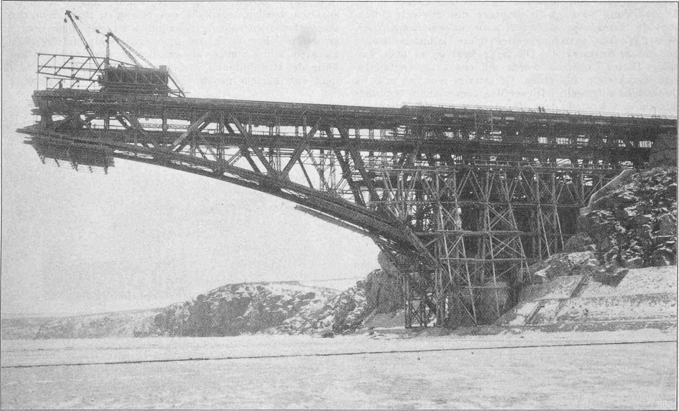
Abb. 18. Freies Vorbauen der Eisenbahn- und Strassenbrücke über den Dnjepr bei Alexandrowsk (Südrussland).
