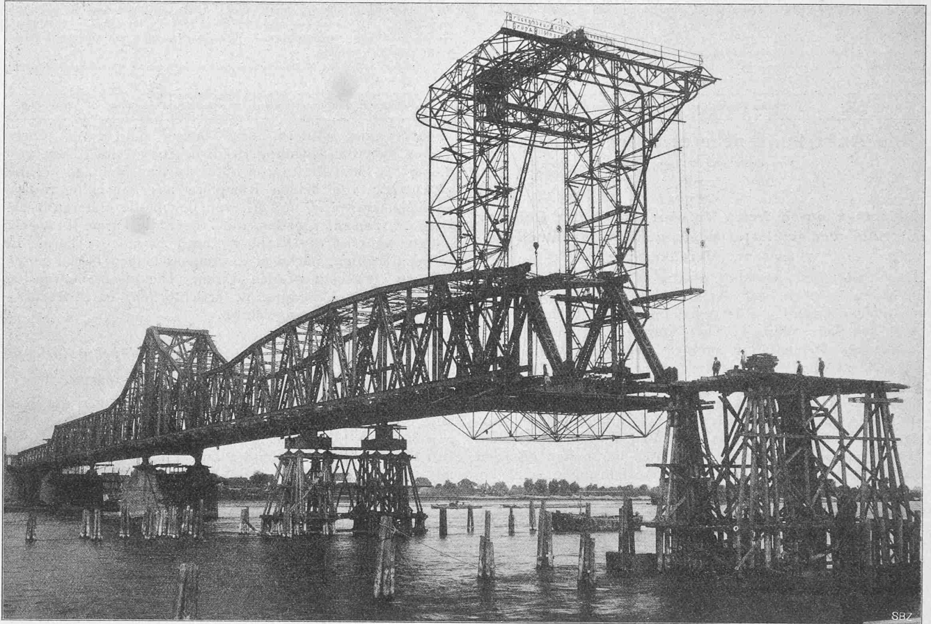
Abb. 16. Freies Vorbauen des mittlern Ueberbaues der Ruhrort-Homberger Strassenbrücke über den Rhein.
