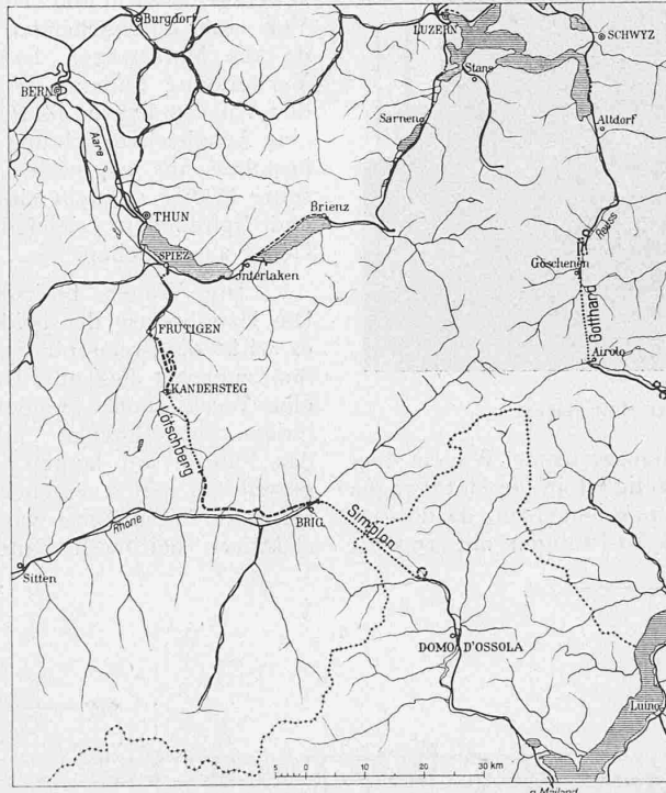
Abb. 1. Uebersichtskarte der Bahnverbindung Bern-Simplon (-Mailand) mit der Strecke Spiez-Frutigen der Lötschbergbahn. — 1:1250000.
