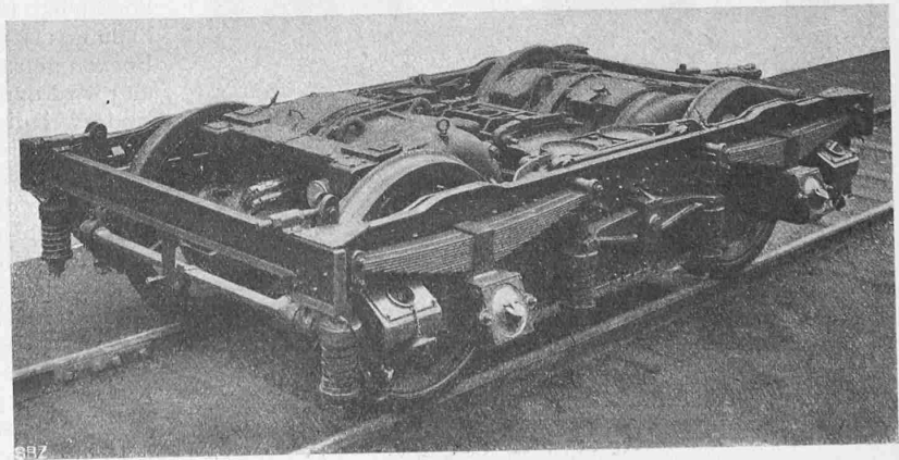
Abb. 7. Draufsicht des Drehgestells zum Motorwagen.
