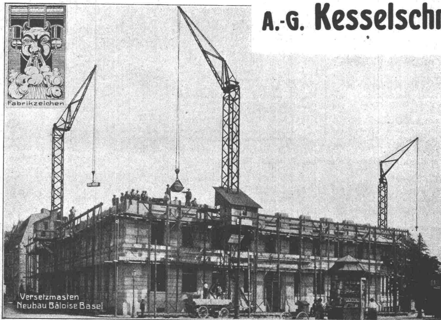
3 Baukranen à 28 m Höhe für 3000 kg. Nutzlast.
