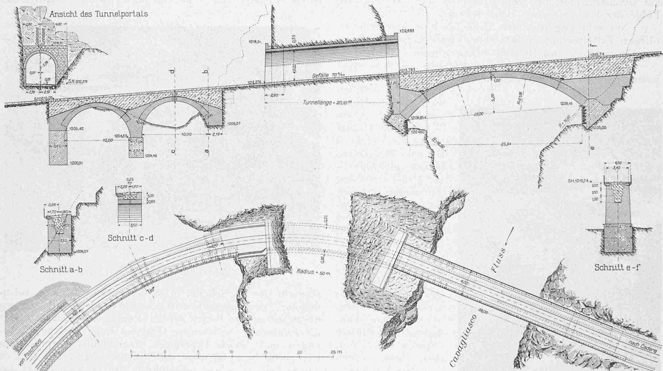
Abb. 44. Lehnviadukt bei Km. 40,8 mit anschliessendem Tunnel und untere Cavagliasobrücke. — Grundriss und Schnitte. — 1:500.
