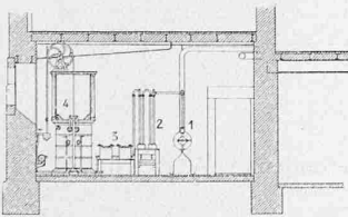
Kleine Versuchsgasanlage
