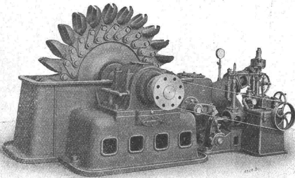
Turbine Pelton de 6300 HP. avec régulateur à double action. 730 mètres de chute, 500 tours par minute.
