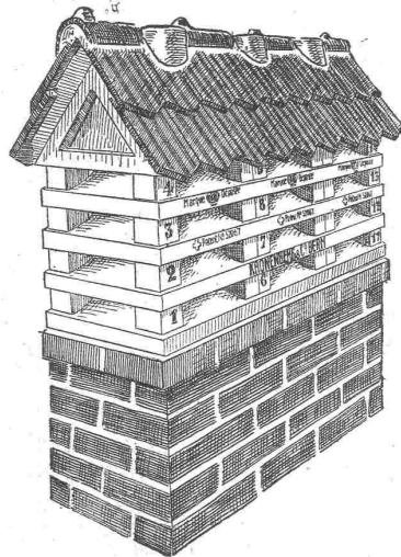
Modell J dreizüig, auch zwei-, vier- und mehrzüig
