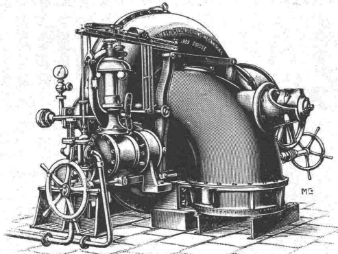
Turbine Francis 900 chevaux, avec régulateur hydraulique.
