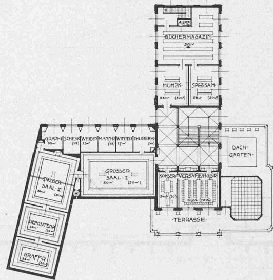
Grundrisse vom Erdgeschoss, Obergeschoss und Dachstock. — Masstab 1:800.
