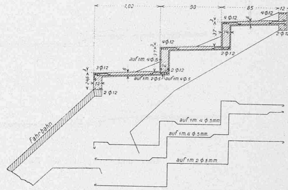
Abb. 11. Armierung der Kurventribünen. — 1 : 50.
