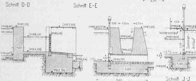
Schnitt G-G
