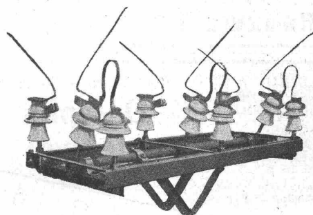
Freileitung-Mastenschalter.
