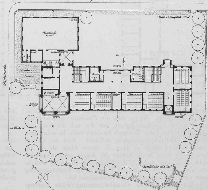
Grundriese und Schnitt. — Masstab 1 : 800.
