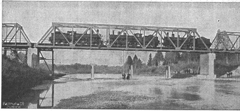
Eisenbahnbrücke über die Thur bei Weinfelden, Linie Wil-Konstanz. Erstellt 1911, Länge 150 m.
