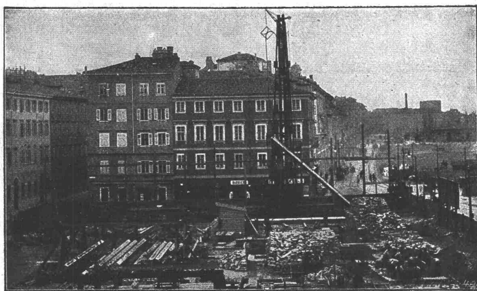
Fundierung des Grand Hôtel Excelsior, Triest mittelst Eisenbetonpfählen, System Züblin. Bild: Bauplatz.
