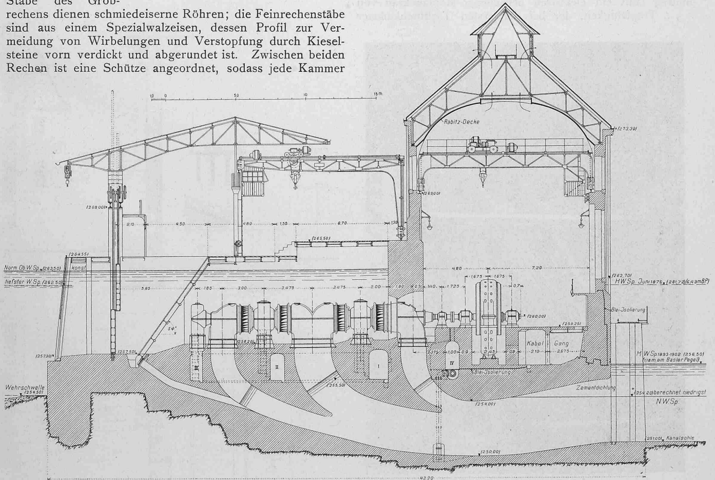
Abb. 5. Querschnitt des Generatorengebäudes mit den Turbinenkammern. — Masstab 1 : 250.
