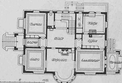
Abb. 1 bis 4. Grundrisse des Landhauses R. Eymann in Langenthal. Masstab 1 : 400.
