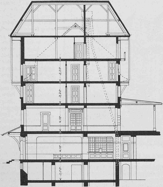
Abb. 7. Querschnitt. — Masstab 1 : 250.
