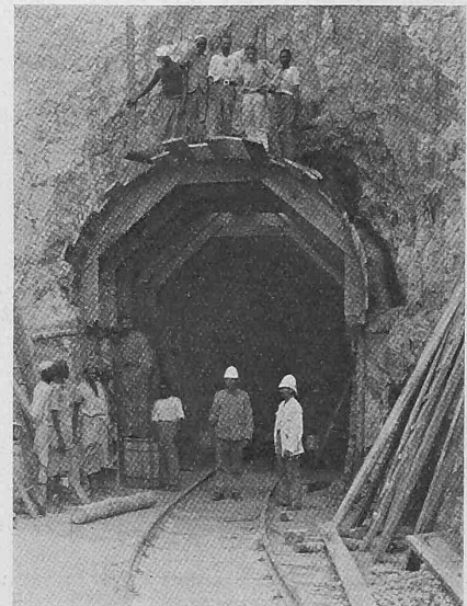
Abb. 14. Tunnelzimmerung bei Km. 21.
