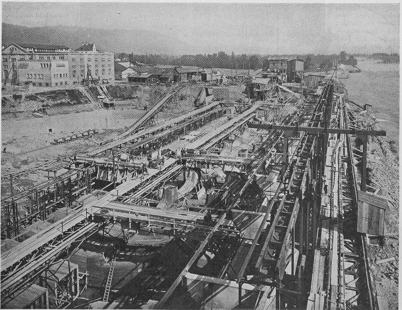
Abb. 84. Baugrube des Unterwasserkanals, Schaung zur Betonierung der Turbinen-Saugrohre (26. IX. 1910).
