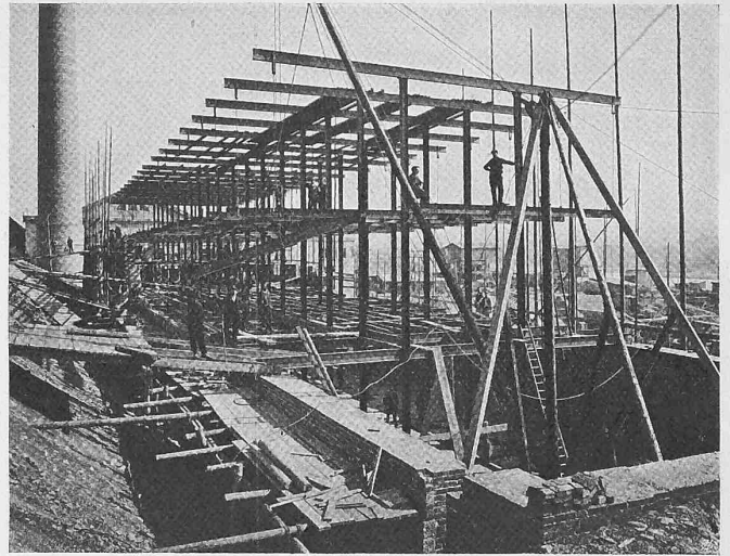
Abb. 85. Eisengerippe des Schalthauses Wyhlen (26. IX. 10).
