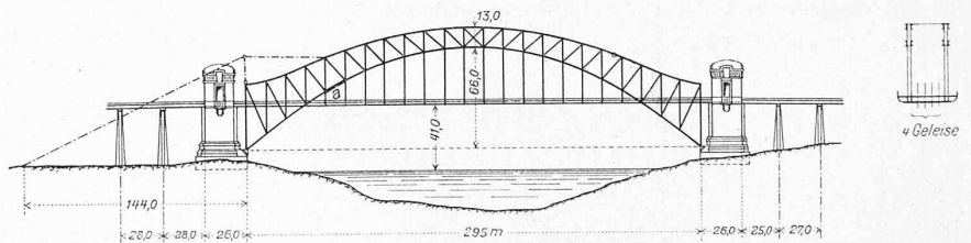
Abb. 52. Hellgate-Brücke über den East-River, New York. — 1 : 5000.
