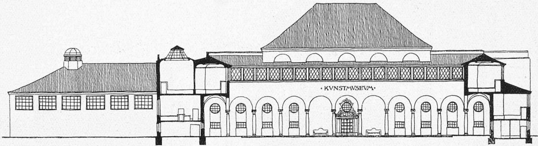
Querschnitt durch den Hof. — Masstab 1:600.
