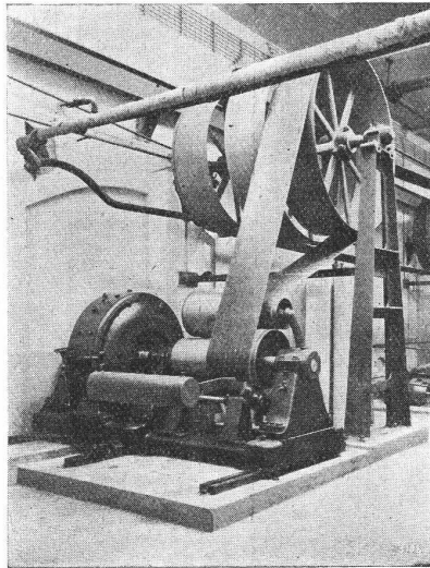
Papiermaschinen-Antrieb mit variabler Umdrehungszahl mit „Stufen-Lenix“ Kraftübertragung 120 PS.
