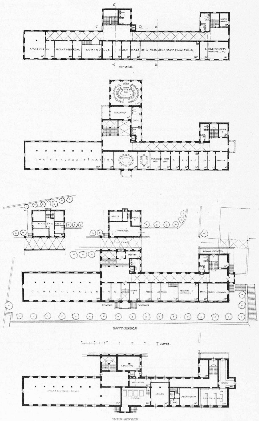
Grundrisse vom Untergeschoss, Hauptgeschoss, I. und III. Stock und Schnitt. — 1:800.
