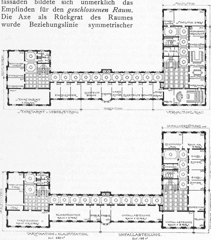
Grundrisse vom II. Stock (unten) und vom III. Stock (oben). Masstab 1 : 800.
