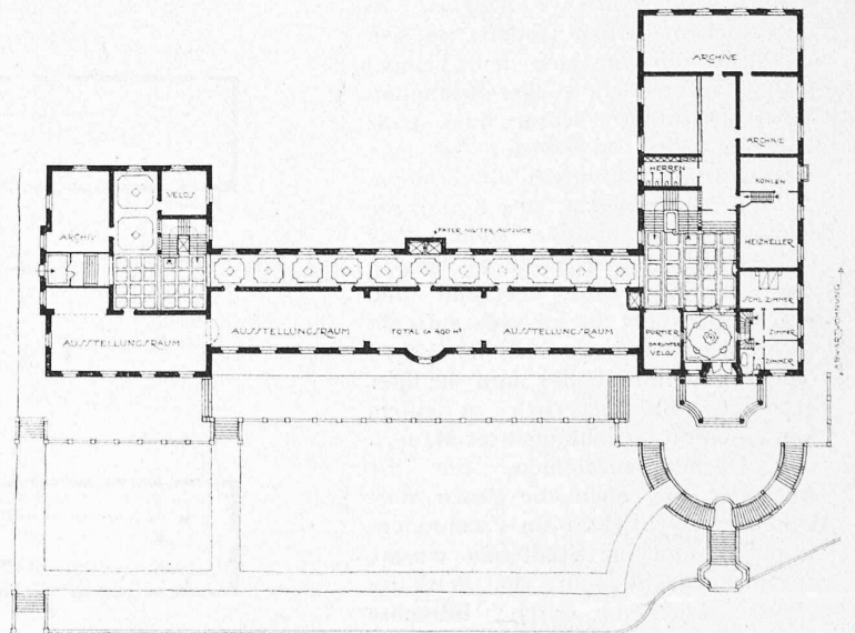
Schnitt und Grundrisse 1: 800. Oben: 1. Stock mit Erweiterung. Unten: Erdgeschoss.
