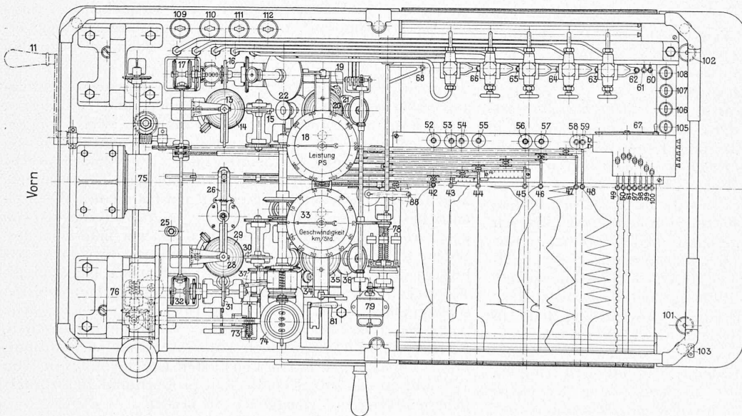
Legende zum Apparatesch des Dynamometerwagens (Abb. 28 bis 32).
