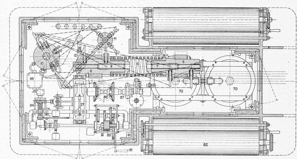
Abb. 32. Horizontalschnitt unterhalb der Tischplatte. — Masstab 1:12,5.
