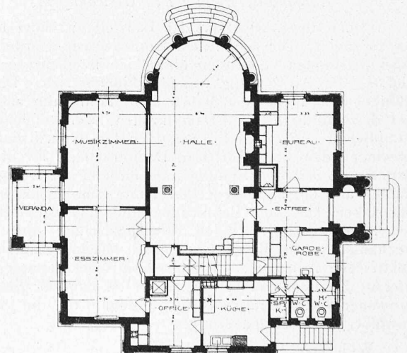
Abb. 1 und 2. Grundrisse vom Keller und Erdgeschoss. Masstab 1:300.
