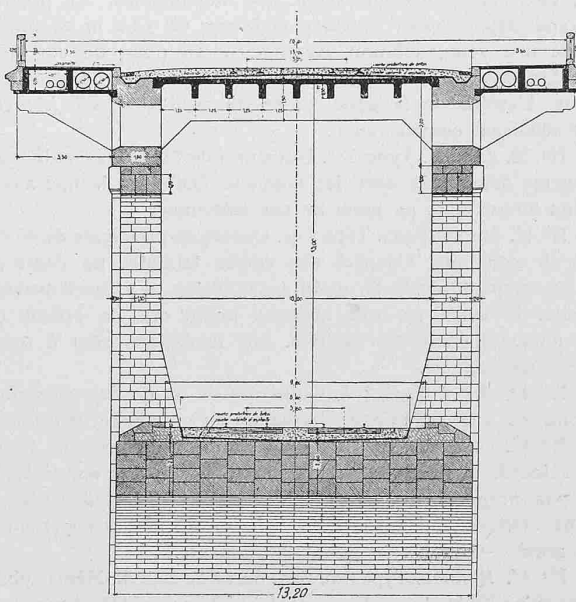
Abb. 8. Nr. 53, Variante B: Eisenbeton-Rahmen-Aufbau.
