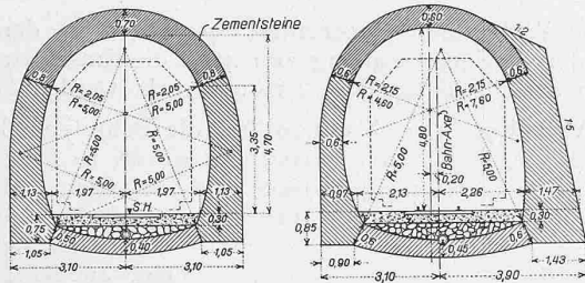
Abb. 20. Spezialprofile Va und VIa. — Masstab 1 : 200. (a in der Geraden, b in Kurven.)
