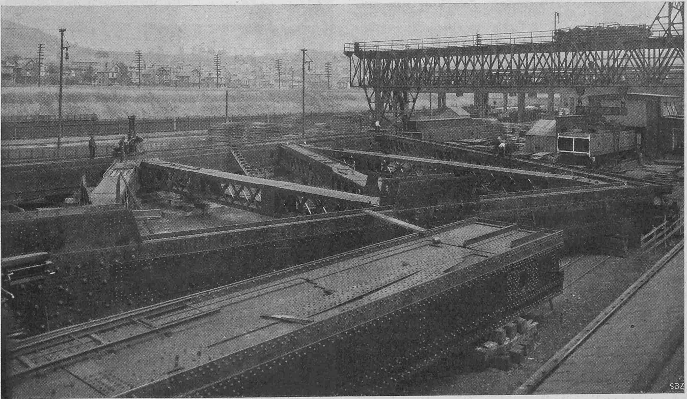
Abb. 5. Zusammensetzen von vier Feldern eines Trägers im Werkhof mit Hülle eines Bockkrans für 150 t Tragkraft bei 40 m Spannweite.
