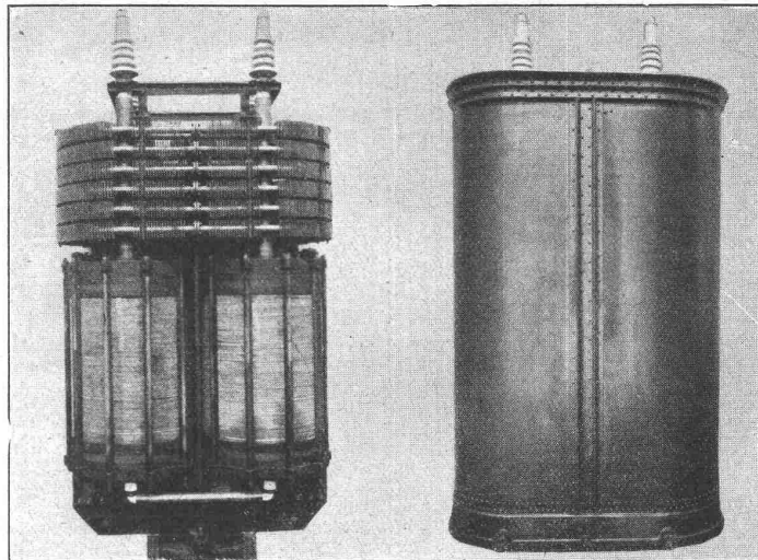
Einphasen-Wechselstrom-Transformator von 2400 kVA, 6000/60000 Volt, 16 2 / 3 Per.
