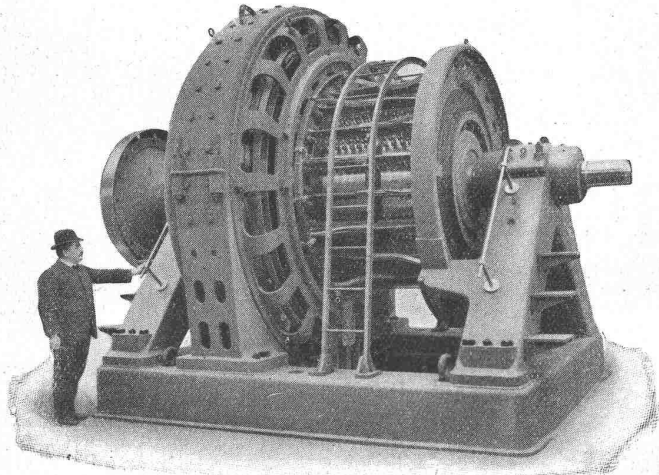
Gleichstromgenerator der Aluminium-Industrie A.-G. Neuhausen, Anlage Chippis, für elektrochemische Zwecke, 3000 kW, 8000 Amp., 375 Volt, 300 Touren per Minute. (Gesamtlieferung: 19 Stück).
