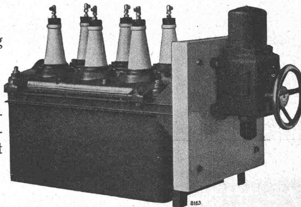
Dreipoliger Hochspannungs-Ölschalter mit Magnet-Fernantrieb
