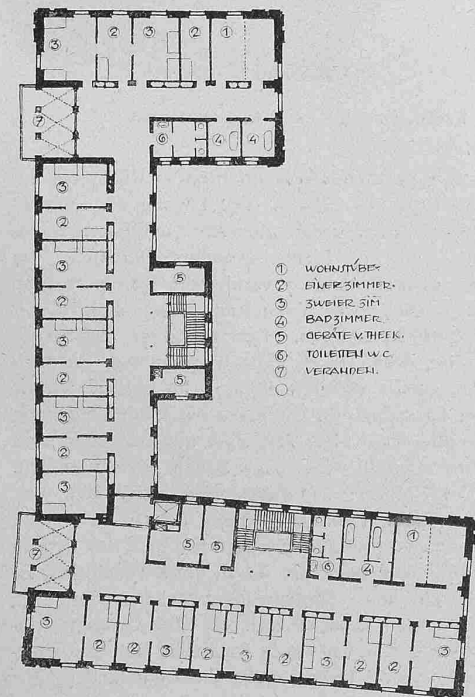
I. Preis, Entwurf Nr. 8. Architekten Möri & Krebs, Luzern. — Obergeschoss 1:600.
