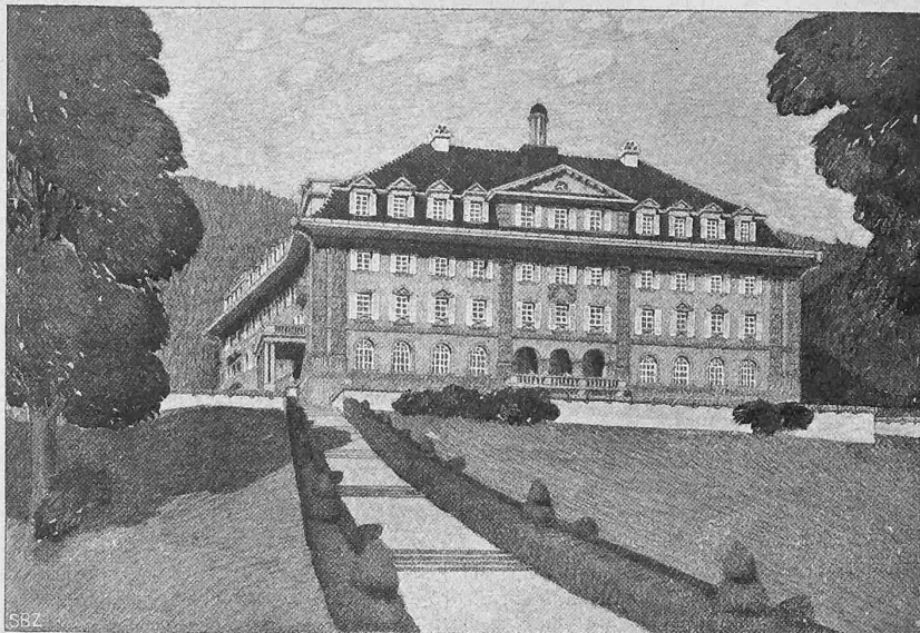
I. Preis, Entwurf Nr. 8. — Architekten Möri & Krebs, Luzern. — Ostansicht.
