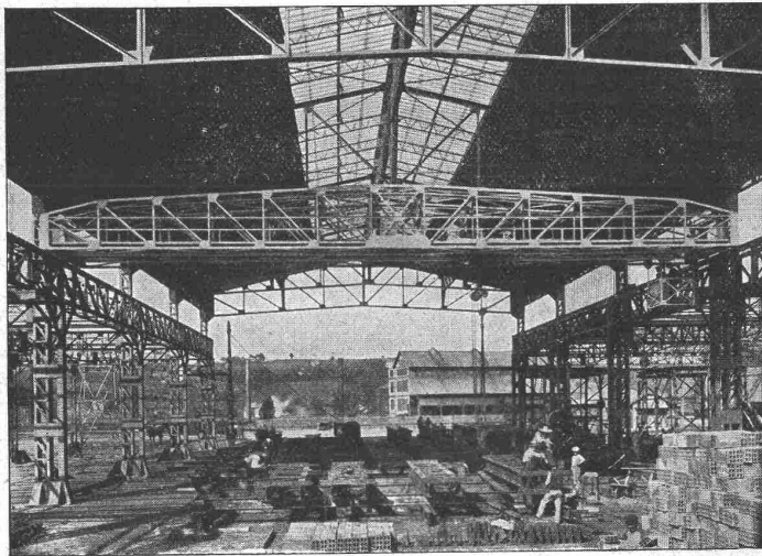
10 Tonnen-Laufkran der Société des Mines de Carmaux in Carmaux.
