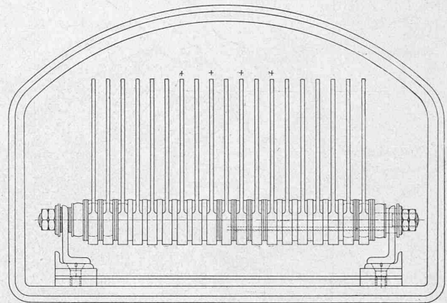
Abb. 2. Querschnitt des Heizkörpers. — Masstab 1:6.
