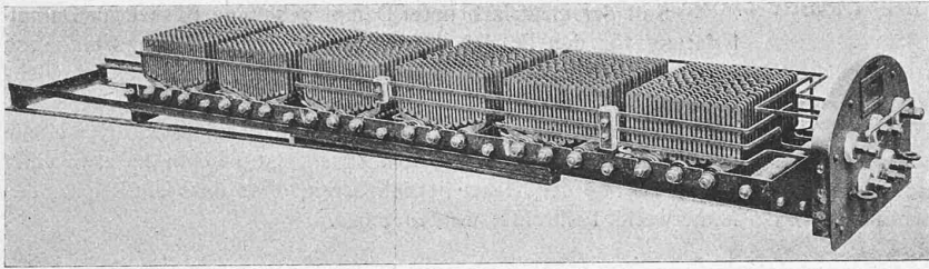
Abb. 1. Elektrischer Kessel-Heizkörper.
