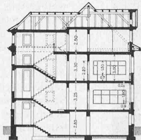
Abb. 8. Schnitt. — 1:400.
