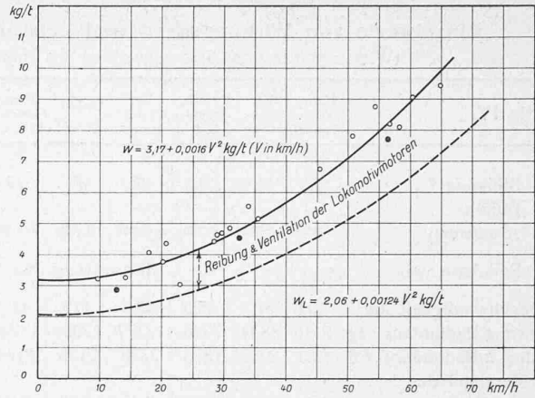
Abb. 7. Rollwiderstand der Lokomotiven 1-E-1 der B. L. S. Gewicht der Lokomotive . . . . . 104,5 t Scheinbares Mehrgewicht der rotierenden Massen . . . . . 44,6 t Für Massenwirkungen einzusetzendes totales Scheingewicht 149,1 t
