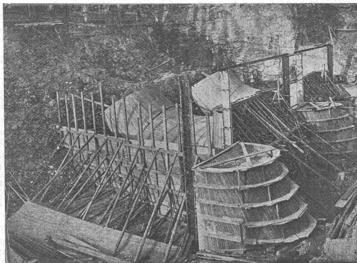
Kraftwerk-Turbinenhaus Olten-Gösgen.
