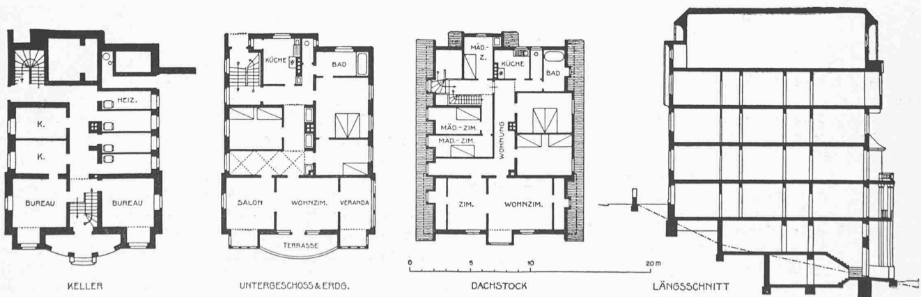
Abb. 1 bis 3. Grundrisse des Mehrfamilien-Wohnhauses Titlisstrasse 58 in Zürich. — Masstab 1:400. — Abb. 4. Schnitt.
