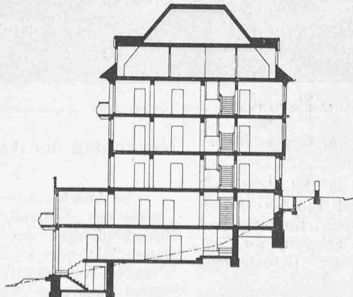
Abb. 9. Querschnitt Titlisstrasse 60. — 1:400.
