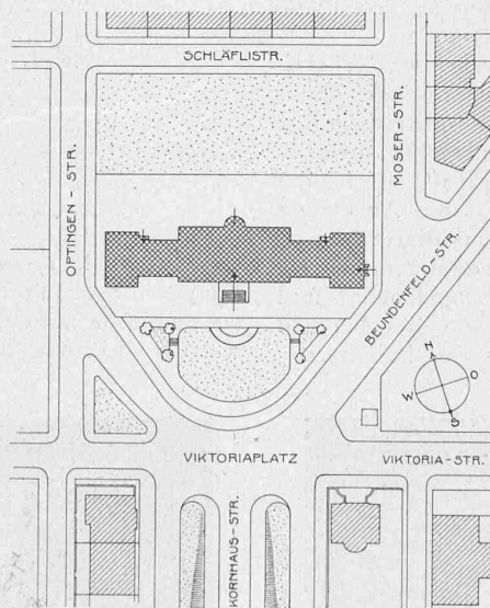
Abb. 1. Lageplan. — Masstab 1:2500.
