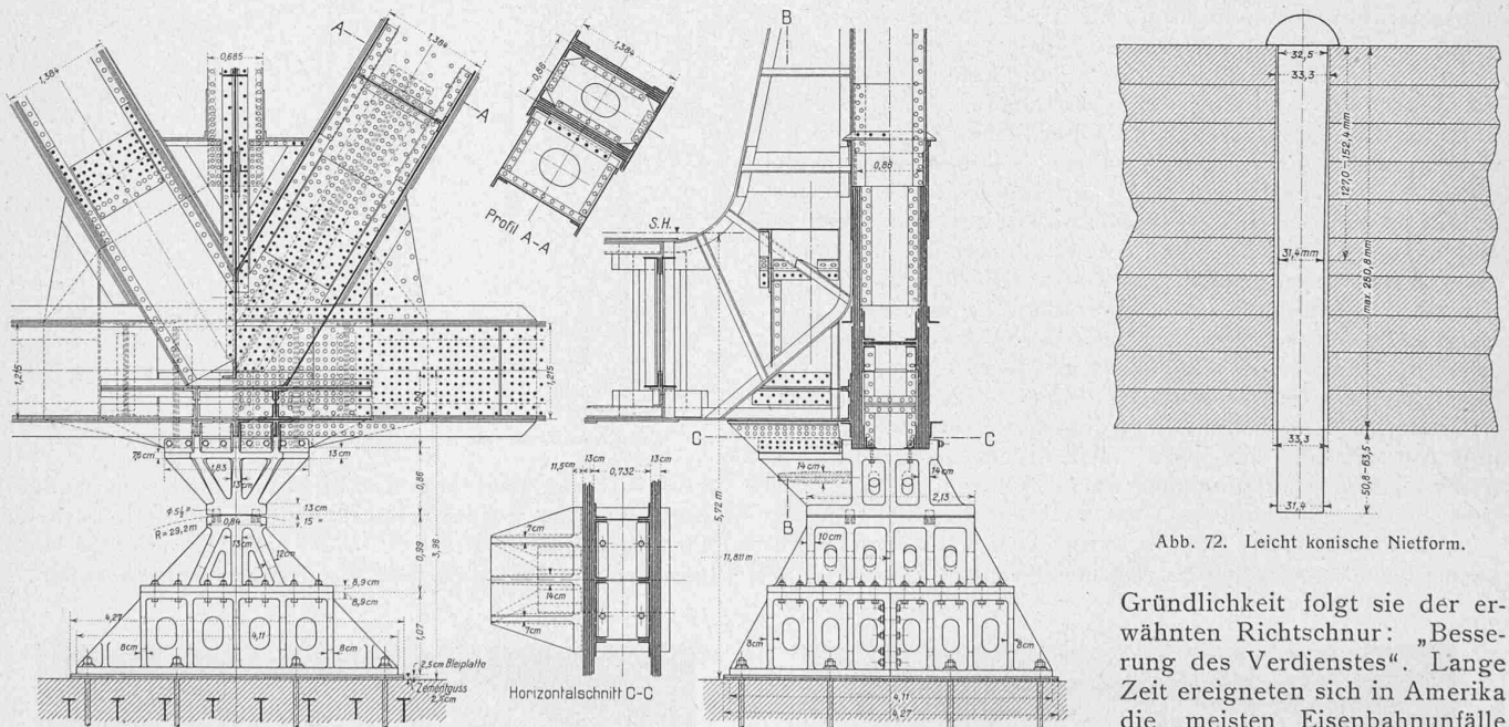
Abb. 71. Auflagerstuhl auf dem Mittelpfeiler der Sciotoville-Brücke über den Ohio. — Masstab 1 : 10.
