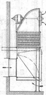
Sendric-Fabrik-Heizapparat mit Frischluftzuführung für Leistungen bis 360000 WE pro Apparat und Stunde.
