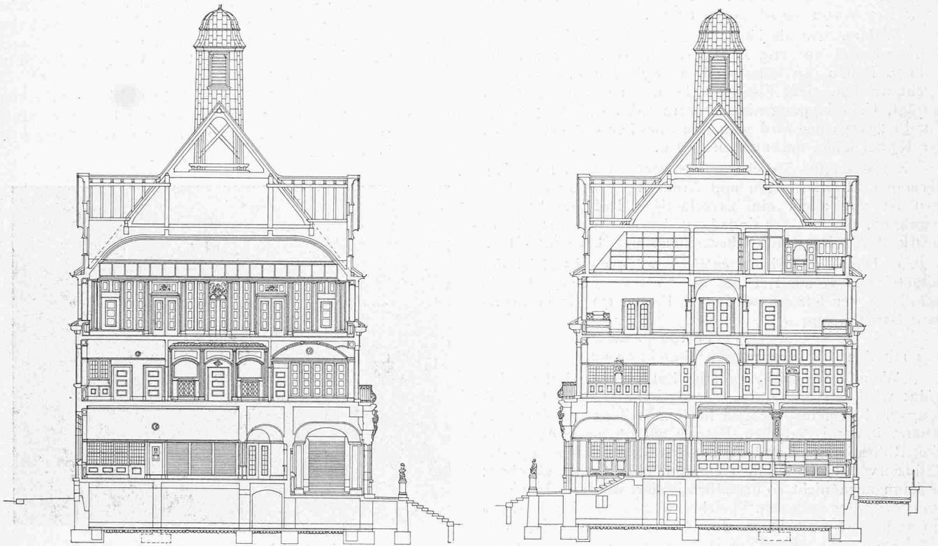
Abb. 11. Schnitt durch Osteingang (Staatsgebäude). — Masstab 1:300. — Abb. 12. Schnitt durch Westeingang (Kantonalbank).
