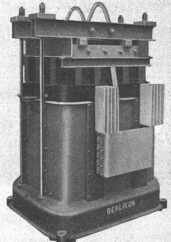
Einphasenwechselstrom-Transformator mit künstlicher Luftkühlung. Leistung 1500 kVA, 4000 Volt primär, 100 Volt und 15000 Ampère sekundär, 50 Perioden.
